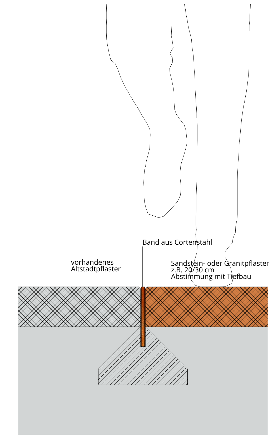
Detail Cortenstahlband M 1:5
